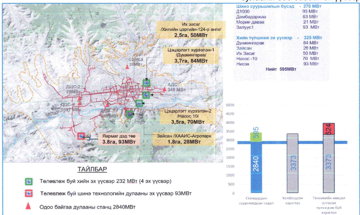
Зураг 33. Дулаан хангамжийн сүлжээнд төлөвлөж буй дулааны бие даасан эх үүсвэр:
